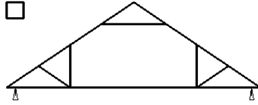
Ferme comble aménageables à entrain porteur
