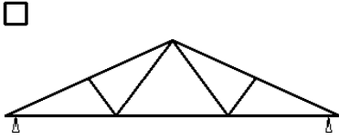
Ferme comble perdus
